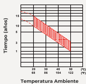
Vida útil (Flotación)
