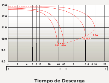
(IV) PARA 12V BATERÍA Tiempo de Descarga VS. Corriente de Descarga (25°C)
