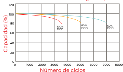
Número de ciclos VS DOD @ 25°C, 0.5C
