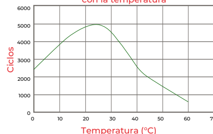
Ciclo de vida en relación con la temperatura
