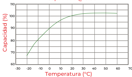
Efecto de temperatura / Capacidad @ 0.5C
