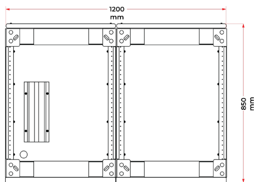
VISTA INFERIOR
