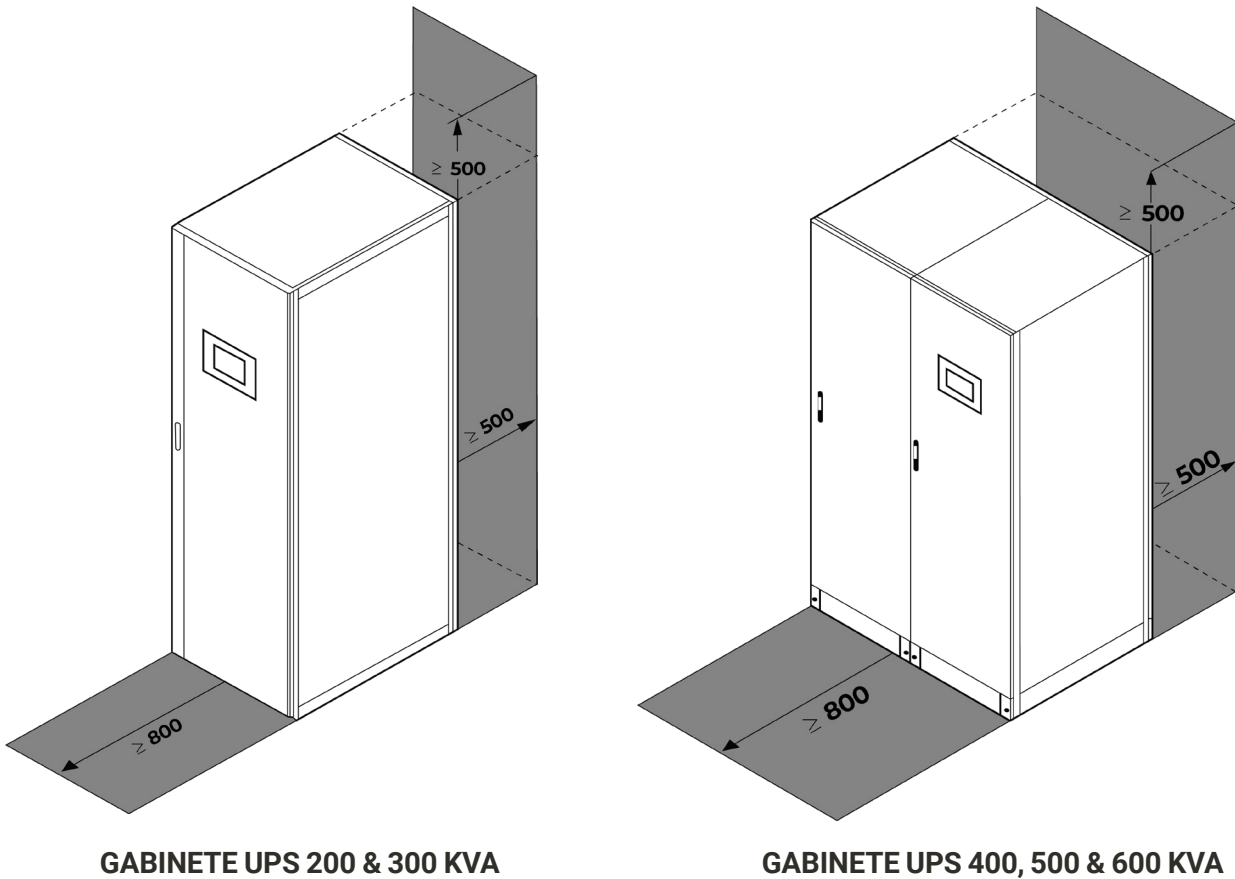
FIGURA 3.1. ESPACIO RESERVADO PARA INSTALACIÓN.
