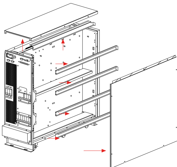
1. DESMONTAR LAS CUBIERTAS Y LOS TRAVESAÑOS.
