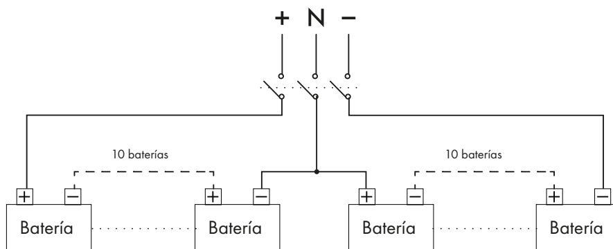
FIGURA 3.7. DIAGRAMA DE BANCO DE BATERÍAS (CADENA)
