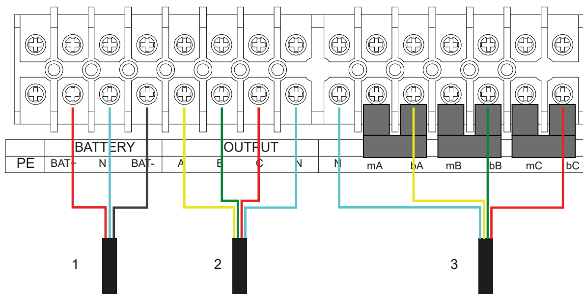
FIGURA 3.6. CABLEADO DE UPS (PS33-10TL & PS33-15TL)
