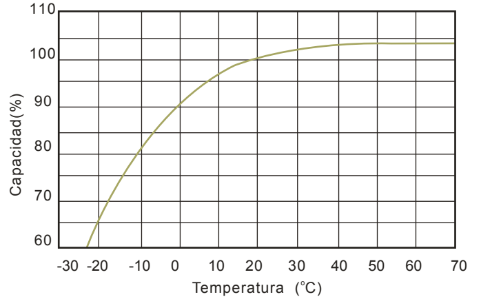
Efectos de temperatura en la capacidad a 0.2C
