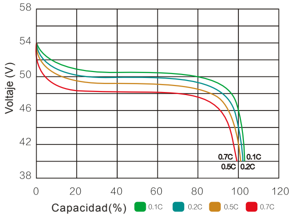
Desempeño en descarga a 25°C
